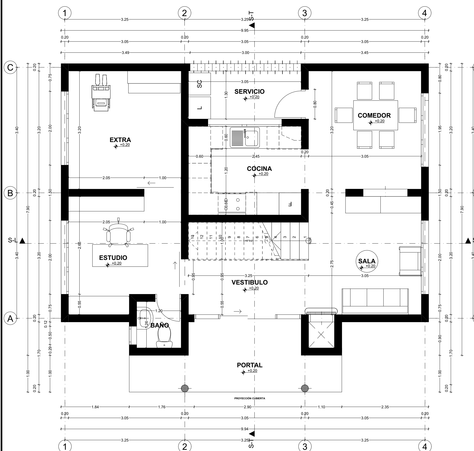
PLANTA BAJA | Esc__1:50
