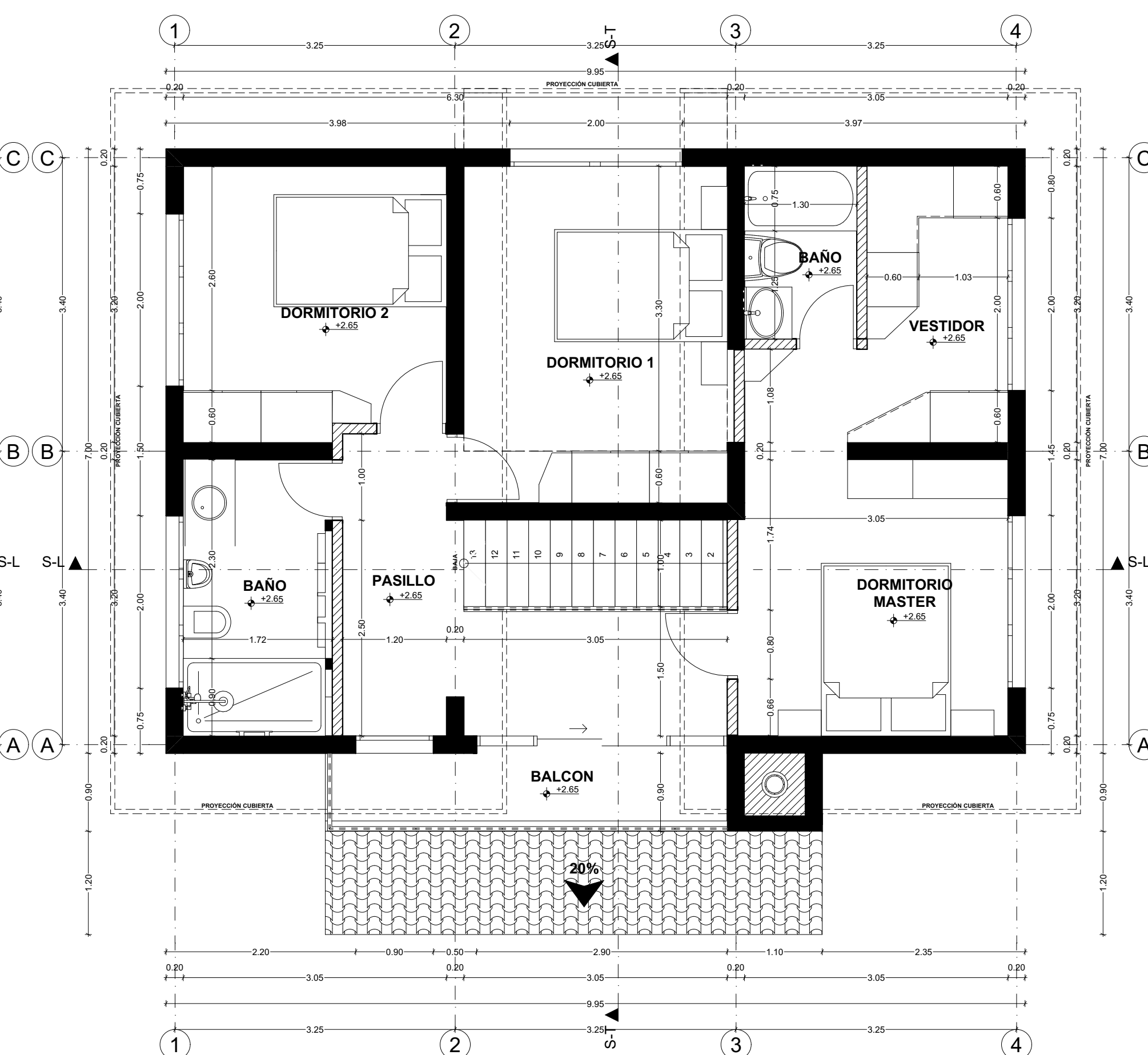
PLANTA ALTA | Esc__1:50
